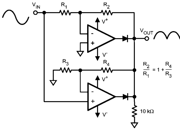
FIGURE 9. Precision Rectifier
